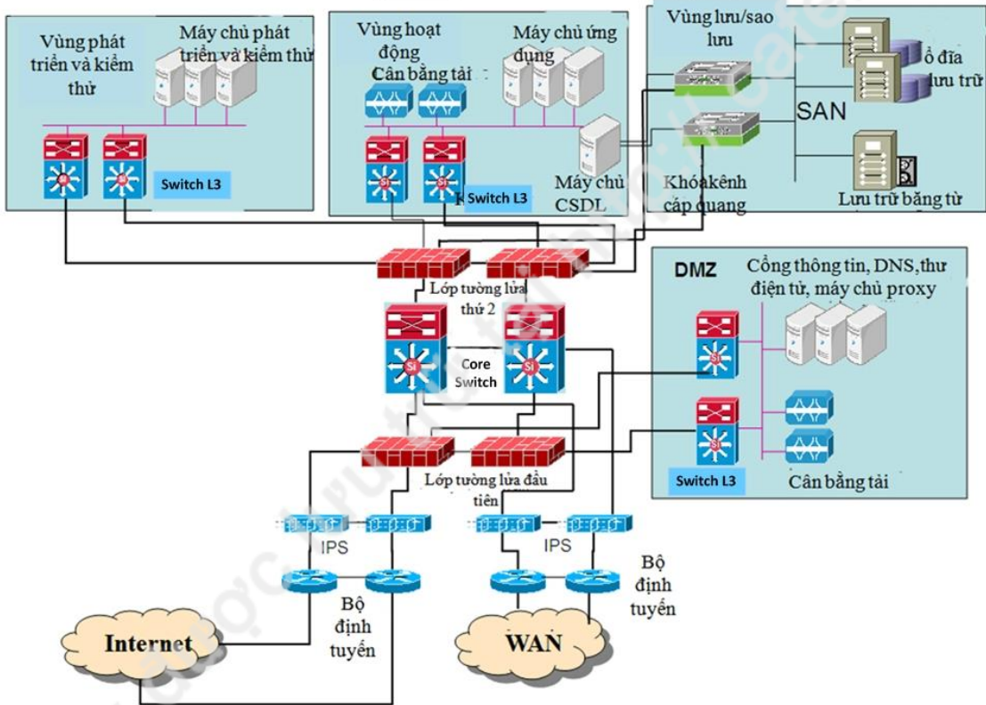
Hình 73: Mô hình triển khai Trung tâm tích hợp dữ liệu Bộ Xây dựng
