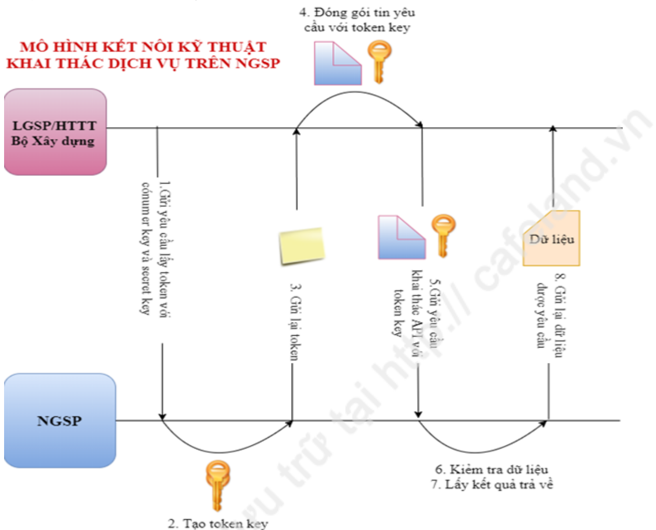
Hình 69: Trình tự kết nối kỹ thuật LGSP và NGSP
