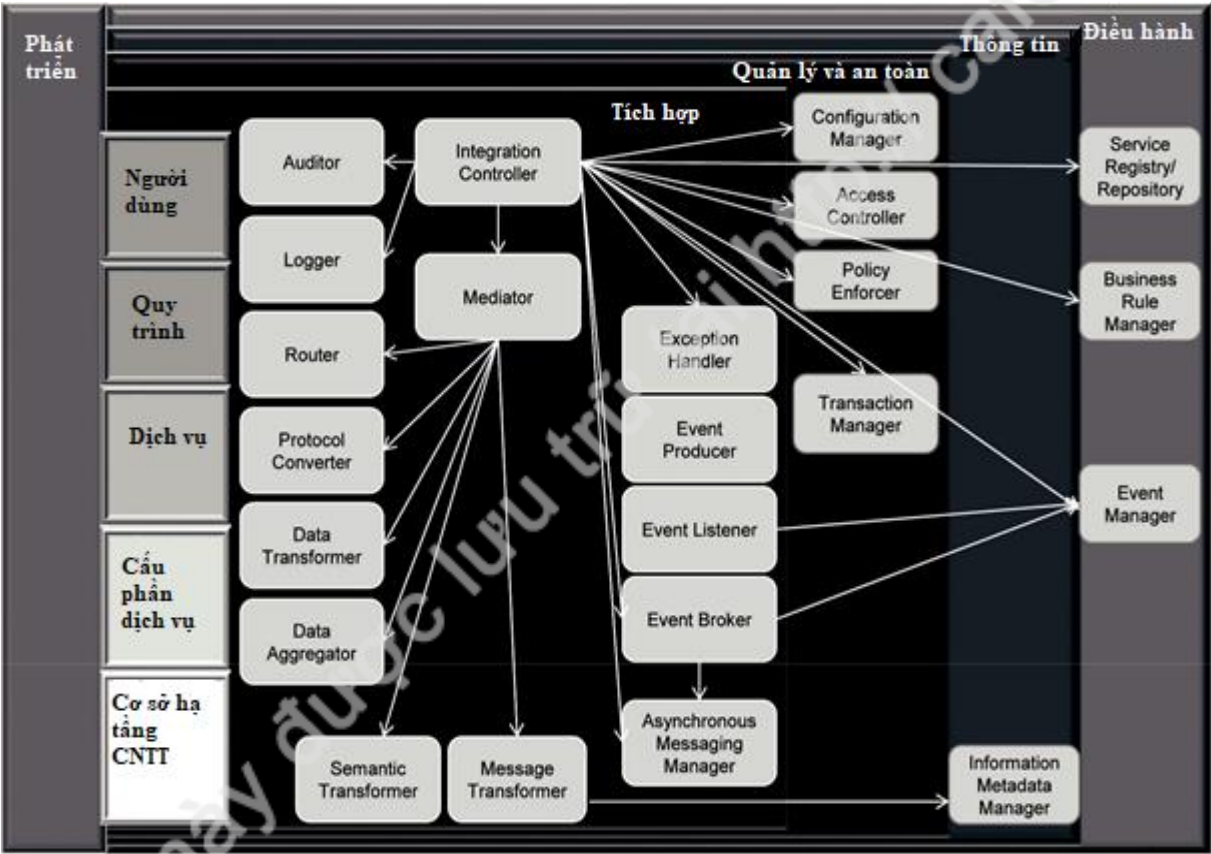
Hình 50: Tương tác giữa lớp tích hợp với các lớp hỗ trợ trong kiến trúc SOA
