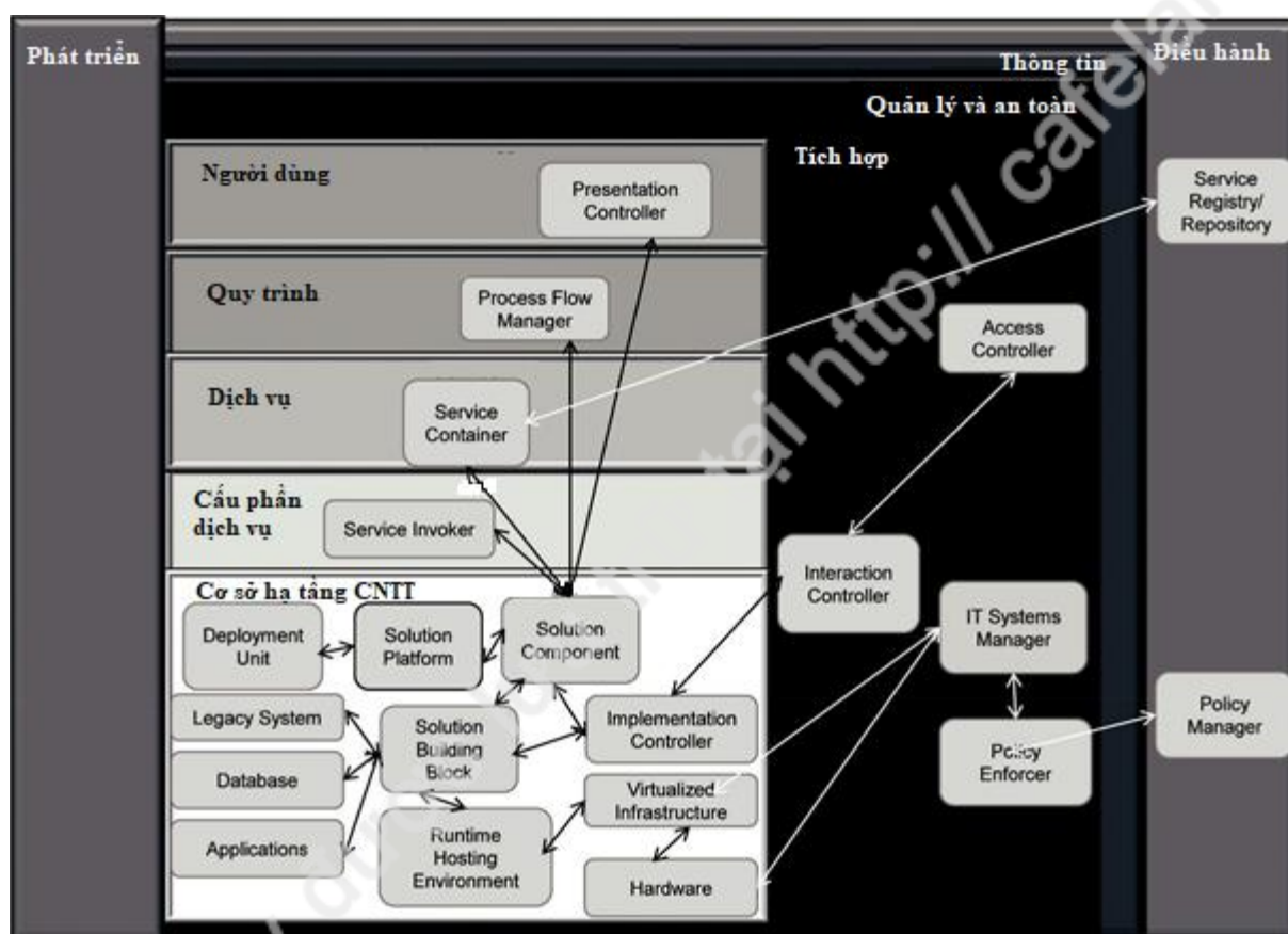
Hình 45 - Các tương tác chính của lớp Cơ sở hạ tầng CNTT với các lớp chức năng
