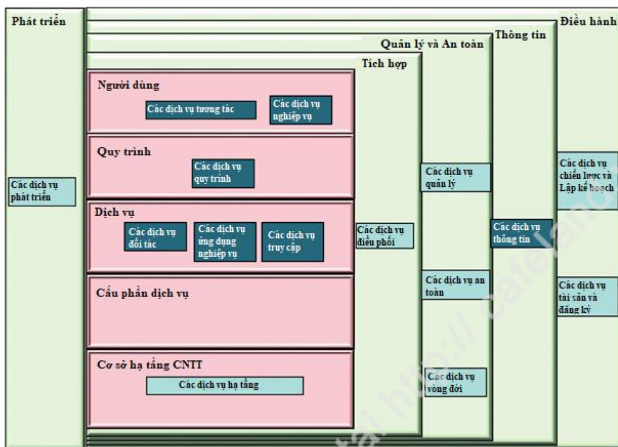
Hình 59: Sự tương đồng giữa các phân nhóm dịch vụ và các phân lớp kiến trúc trong kiến trúc tham chiếu SOA
