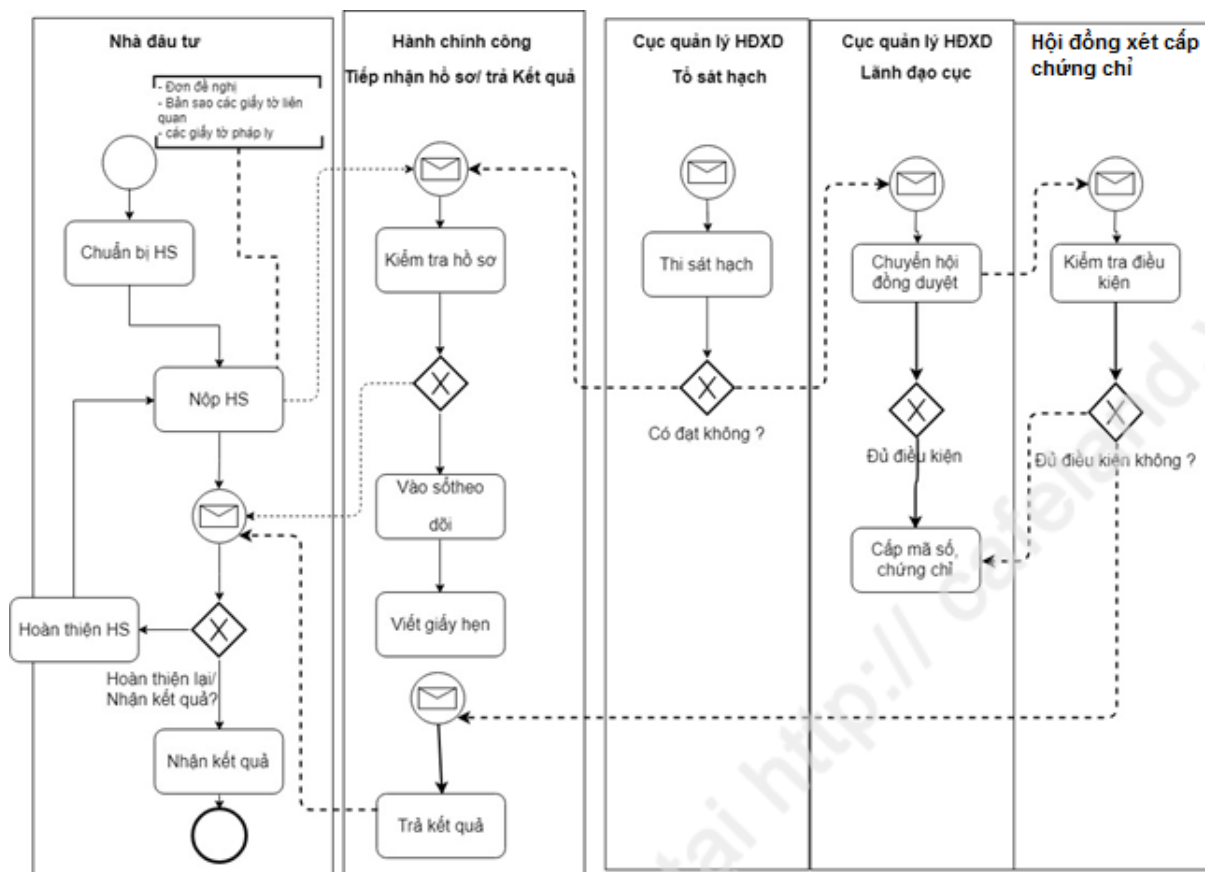
Hình 8: Quy trình nghiệp vụ hiện tại thủ tục Cấp chứng chỉ hành nghề hoạt động xây dựng hạng I đối với cá nhân hoạt động xây dựng trong các lĩnh vực: Khảo sát xây dựng; Thiết kế quy hoạch xây dựng; Thiết kế xây dựng công trình; Giám sát thi công xây dựng; Kiểm định xây dựng; Định giá xây dựng.
